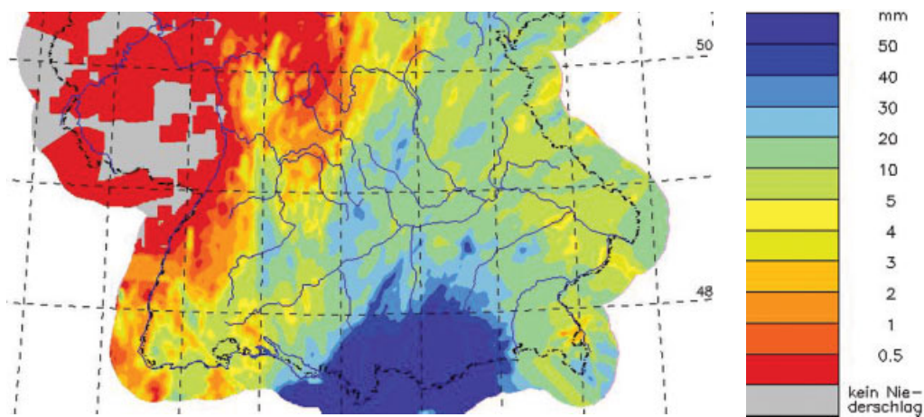
Bild 7. Kombination von Radar- und Stationsdaten für den 22. 8. 2005
