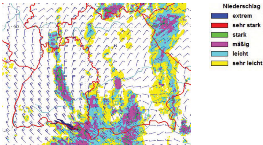
Bild 1. Bodennahes Radarbild (Zentraleuropäisches Kompositbild) und analysiertes Windfeld in 1500 m Höhe NN (LM, 850 hPa) für den 23. 8. 2005, 02 Uhr MESZ
