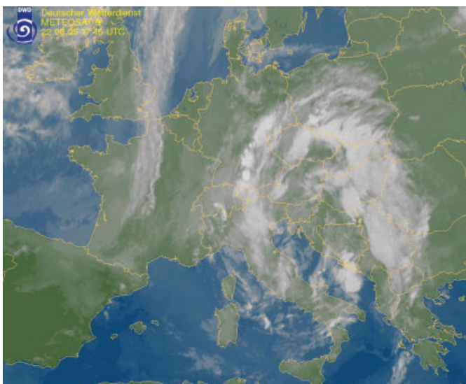
Bild 5. Satellitenaufnahme des METEOSAT 8 für den 22.8.2005, 19.45 Uhr MESZ
