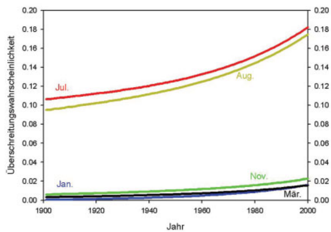
Bild 11. Überschreitungshäufigkeitshäufigkeit des 95-Perzentils für die Station Marktoberdorf (Oberallgäu)
