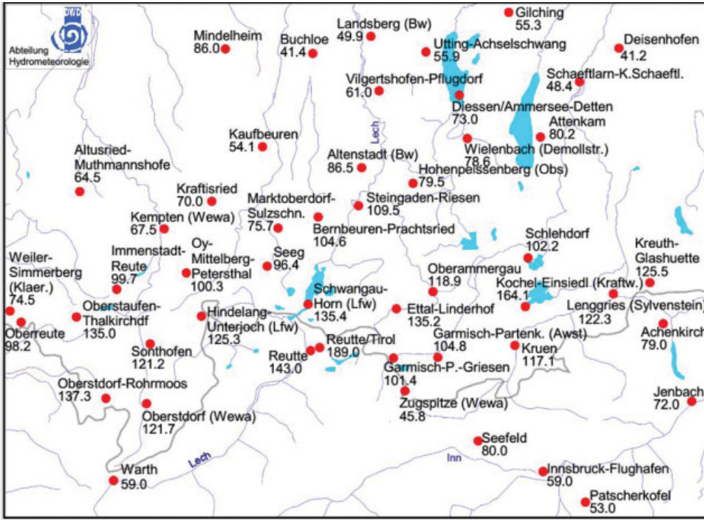
Bild 8. Messwerte der täglichen Niederschlagshöhe in mm (22.–23.8., je 08 Uhr MESZ)
