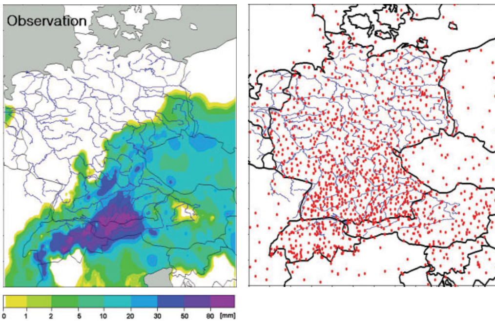
Bild 4. Analyse auf der Basis der Beobachtungsdaten (Messnetze) für den 22.–23.8., je 08 Uhr MESZ, die Lage der verwendeten 1377 Stationen sowie die Legende aller Niederschlagskarten (Bild 2 bis 4, mm pro Tag)
