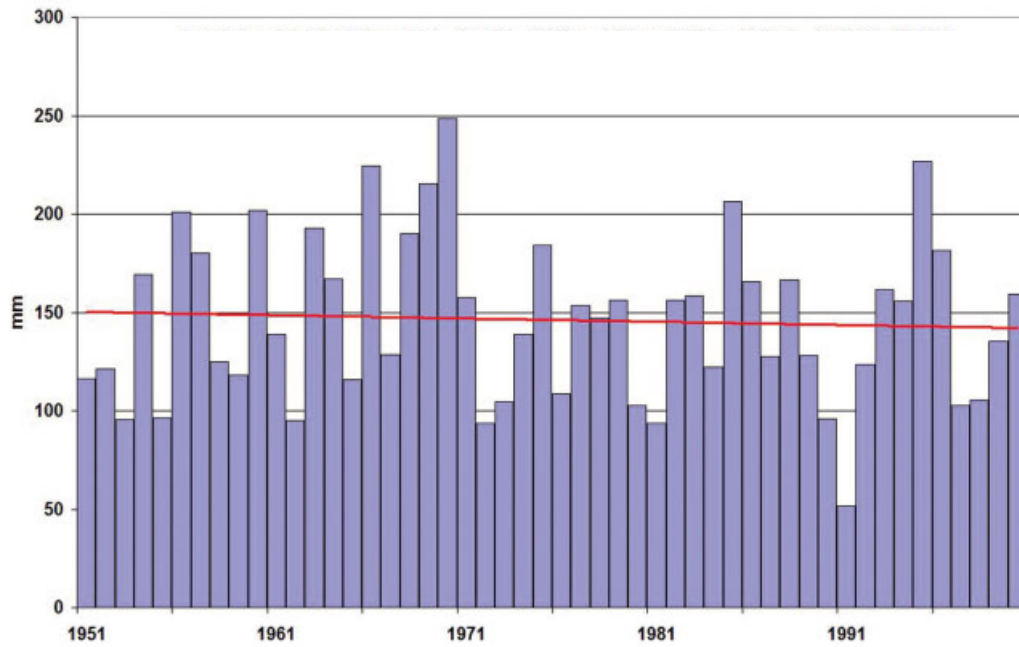
Bild 10. Zeitreihe der monatlichen Gebietsniederschlagshöhe im August für die Region „mittlere Nordalpen“ (9,0°E-12,0°E, 46,5°N-48,0°N)
