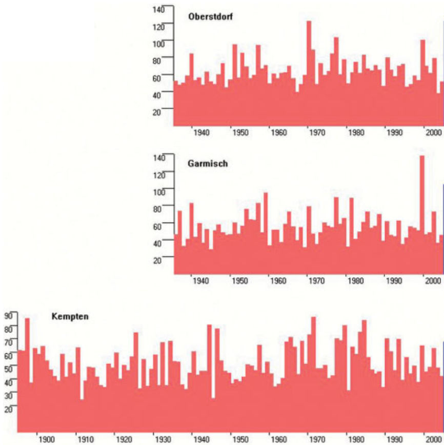
Bild 9. Zeitreihen des an der Station je Jahr höchsten gemessenen Tagesniederschlags in mm für die Stationen Oberstdorf, Garmisch und Kempten
