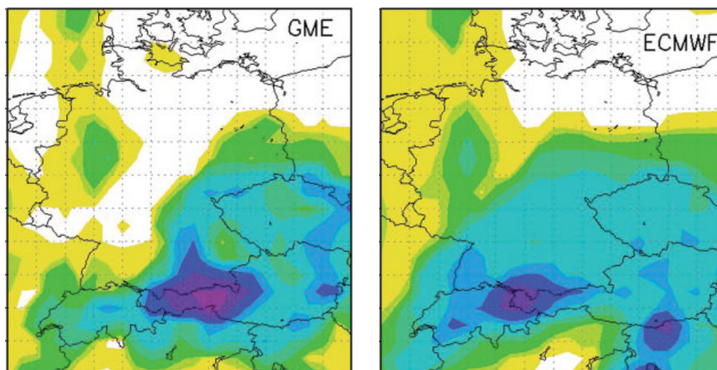
Bild 2. Niederschlagsvorhersagen vom 21. 8. 2005, 02 MESZ, für den 22.–23. 8., je 08 Uhr MESZ
