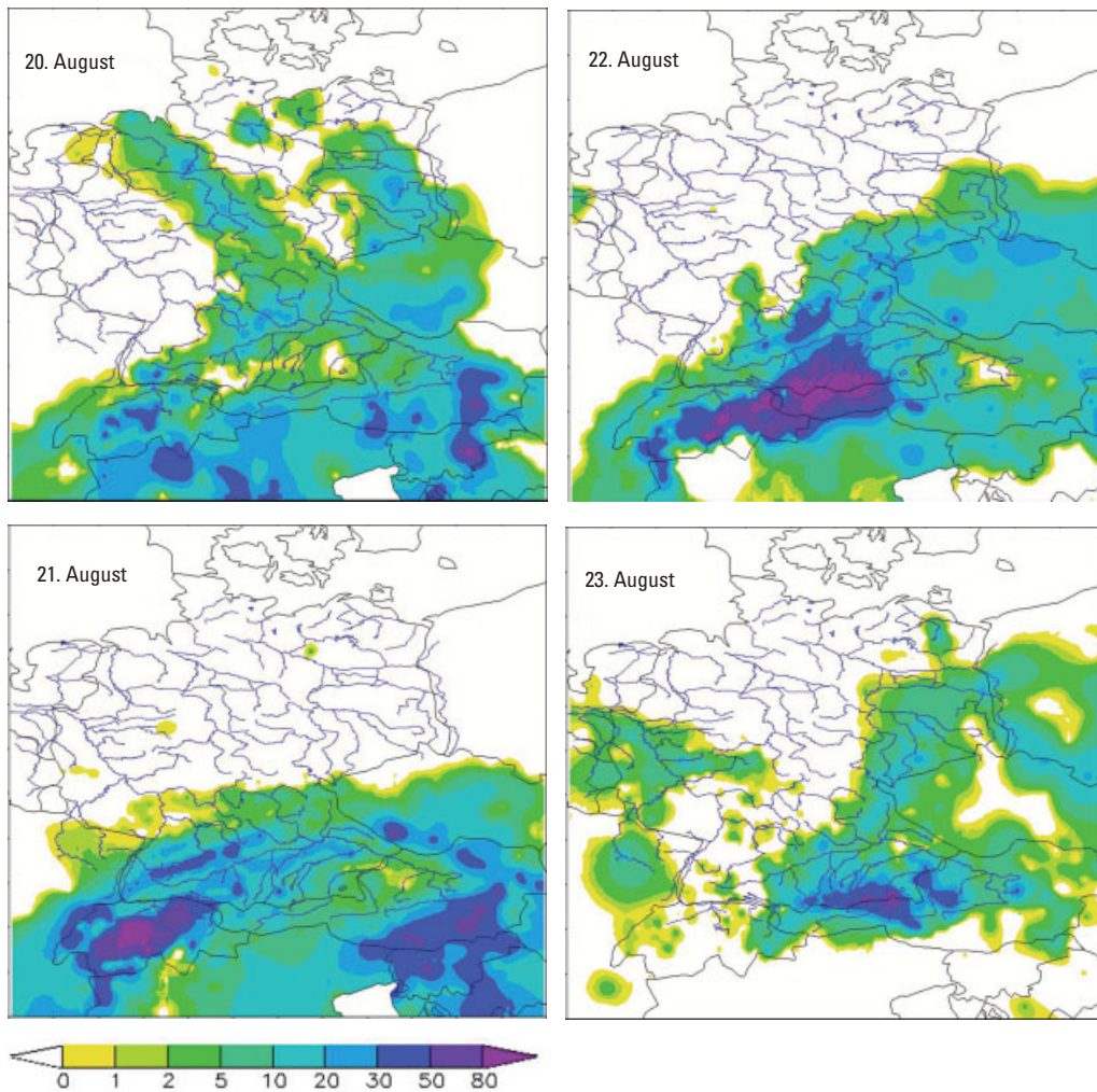
Bild 6. Analysen der Beobachtungen der synoptischen Messnetze des DWD und der Nachbarstaaten für die Episode 20. bis 23. August (jeweils 08 bis 08 Uhr MESZ), Legende: tägliche Niederschlagshöhe in mm ( l/m^2 )
