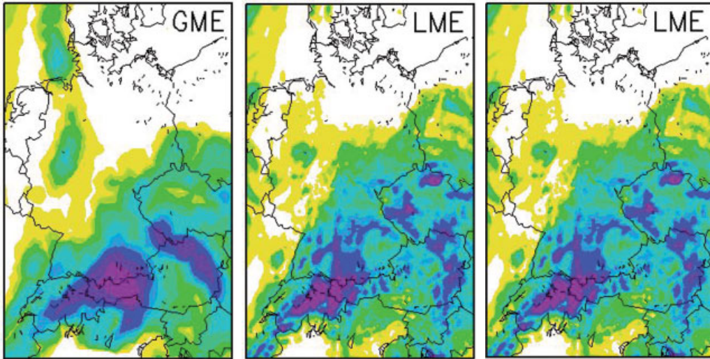
Bild 3. Niederschlagsvorhersagen vom 22. 8. 2005, 02 MESZ, für den 22.–23.8., je 08 Uhr MESZ
